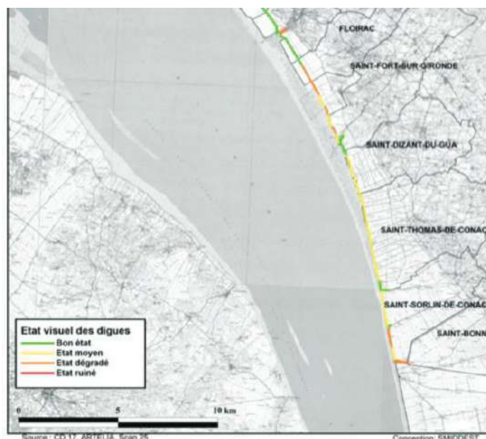
Figure 56 : Etat des digues en Charente-Maritime
