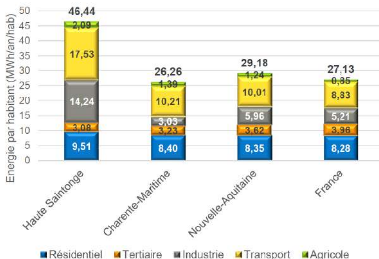
Figure 77 : Consommation d'énergie finale par secteur et par habitant sur le territoire de la Haute-Saintonge
